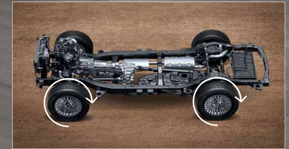
Electric Differential Lock – Front and Rear ระบบล็อกเฟืองขับแบบไฟฟ้าด้านหน้าและด้านหลัง
